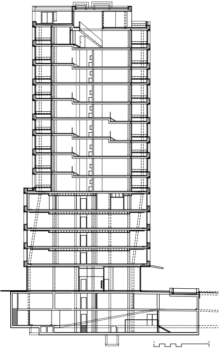
Längsschnitt | Coupe longitudinale
