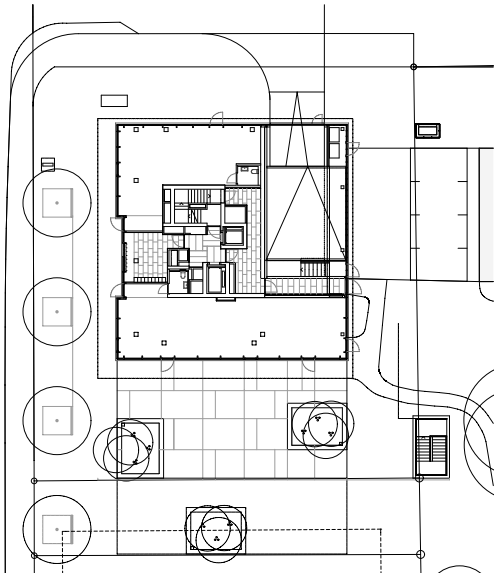
Grundriss Erdgeschoss | Plan du rez-de-chaussée
