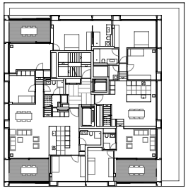
Grundriss 13. Obergeschoss | Plan du 13ème étage
